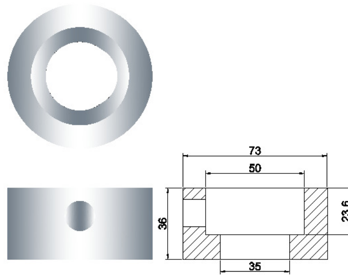
GKMIS_7/1507 5 - 10 DIE HOLDER / SLEEVE
