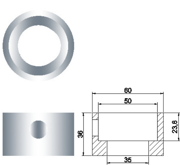
GKMIS_7/1505 5 - 8 DIE HOLDER / SLEEVE
